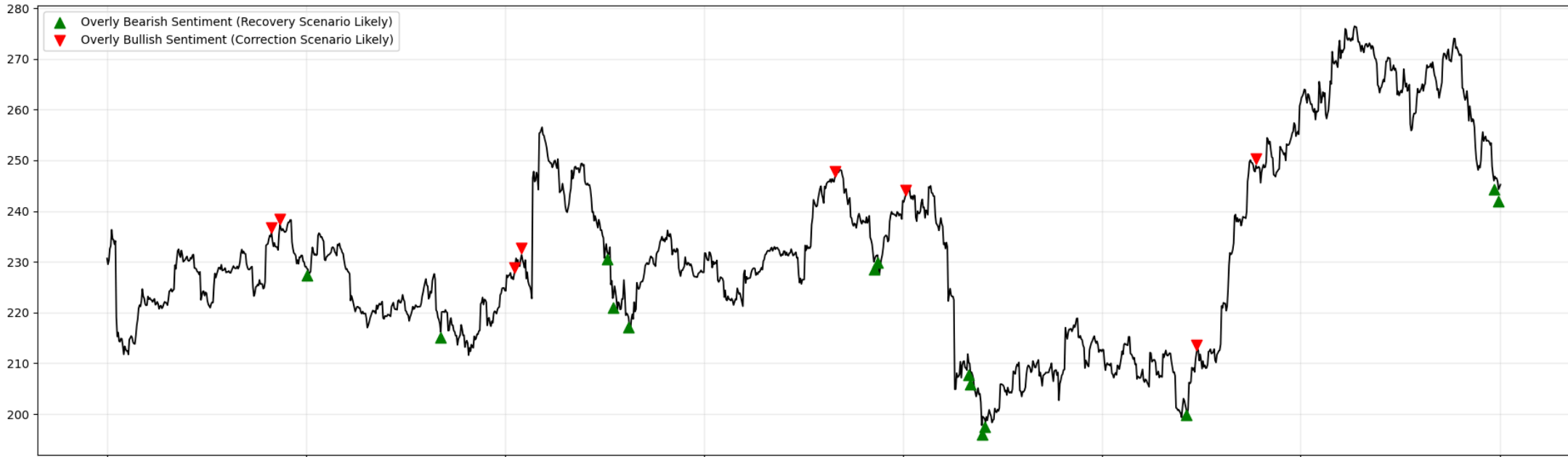
Nexus score
