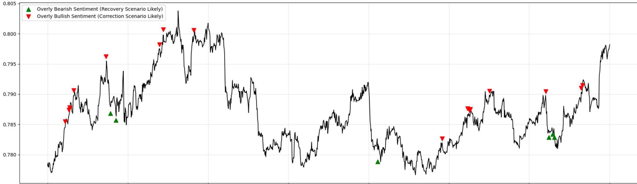
Nexus score
