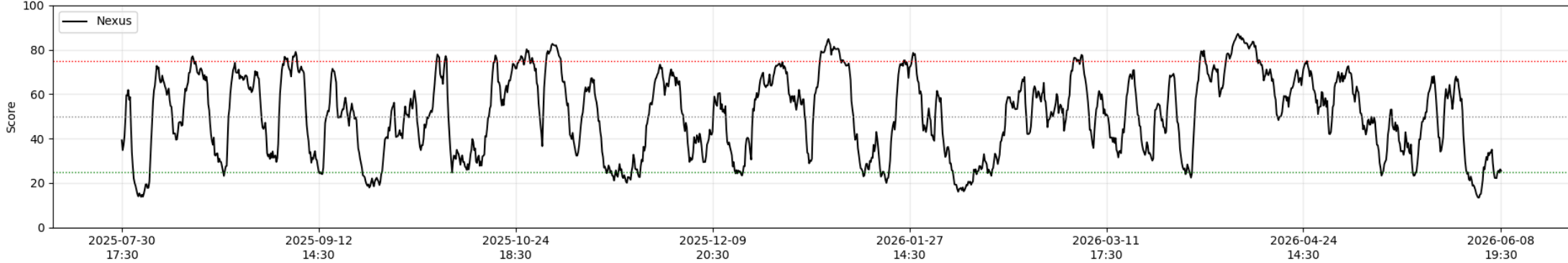
Nexus score
