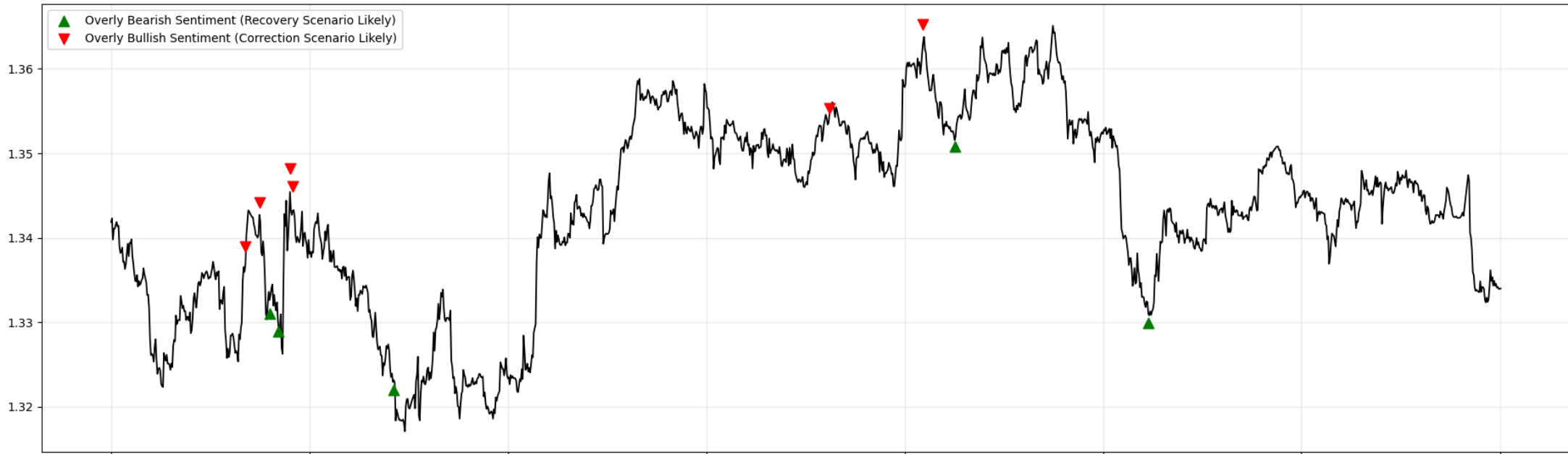
Nexus score
